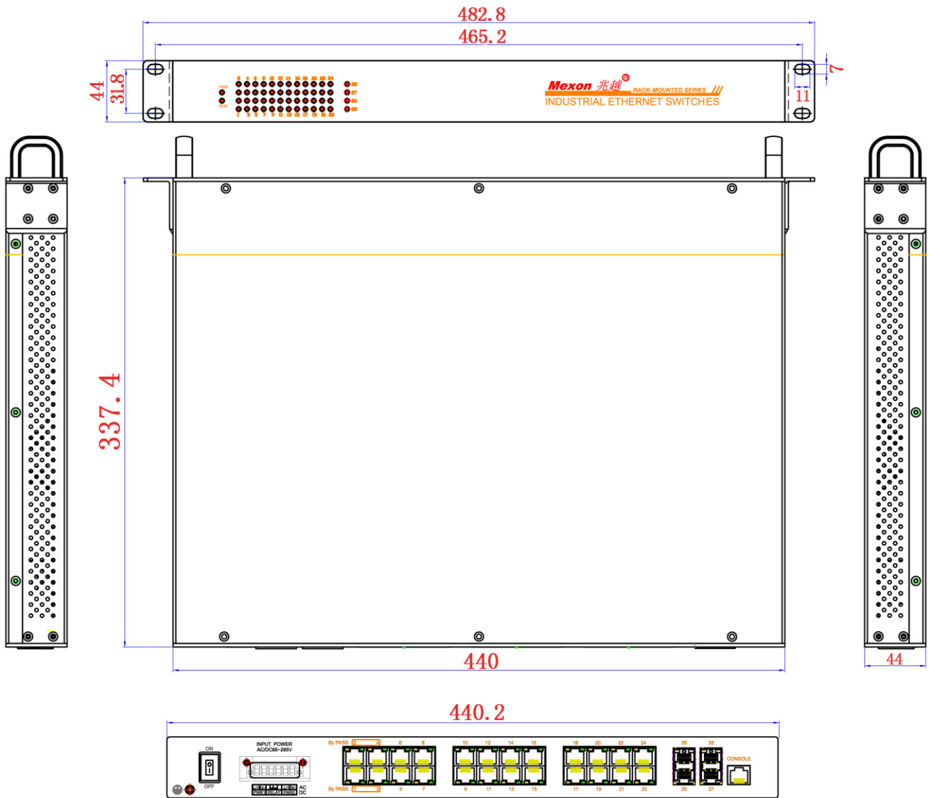
MIER-2428A_P 安装图
