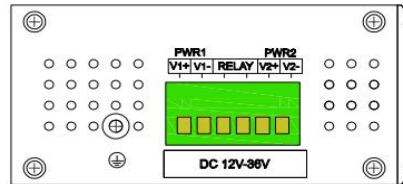
24V电源示意图
