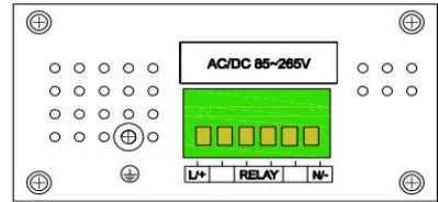
220V电源示意图
