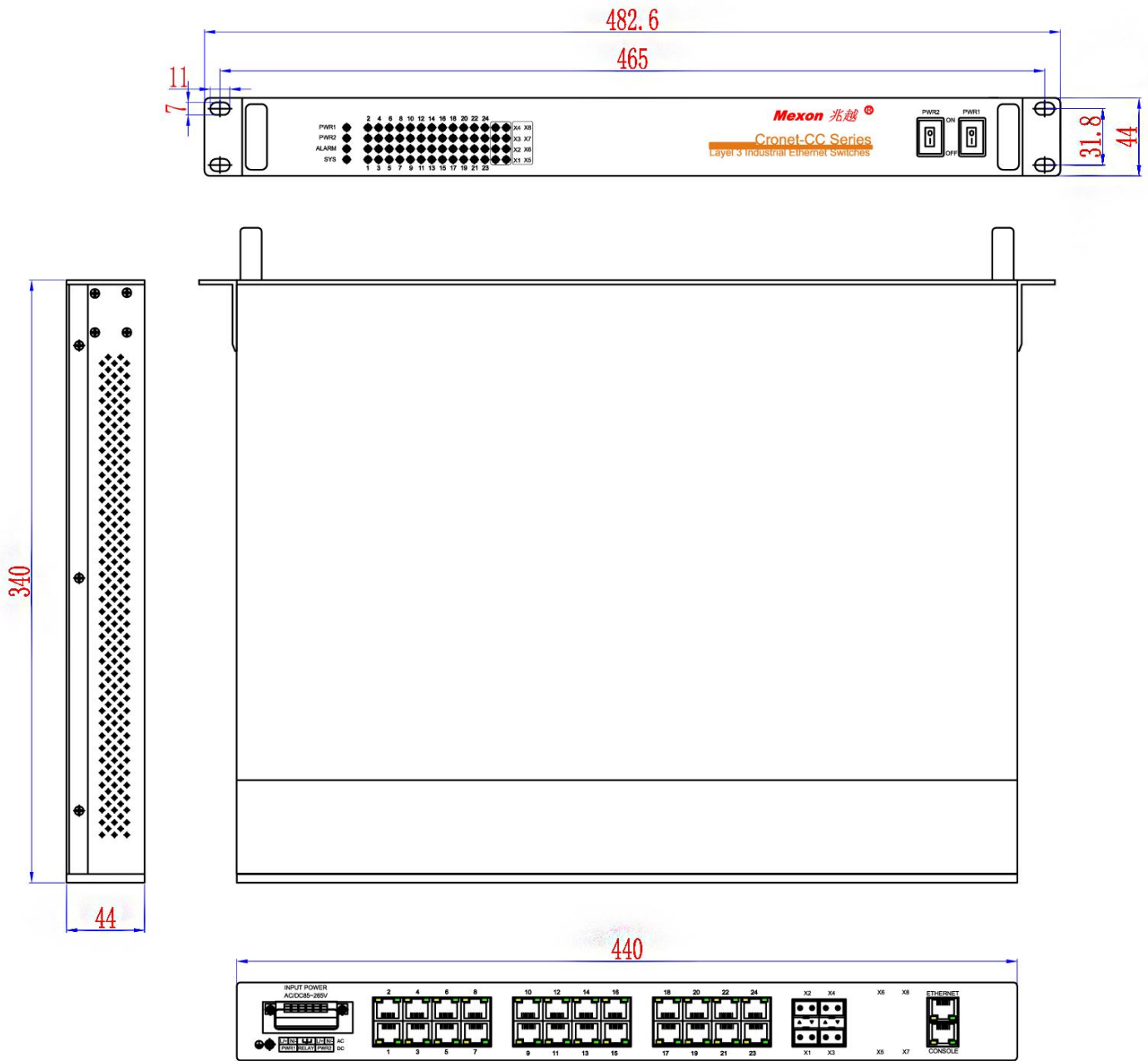
3928 TX4 安装图
